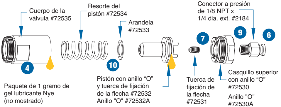
Ensamblaje de pistón, diafragma y flecha para la 725HF-SS
